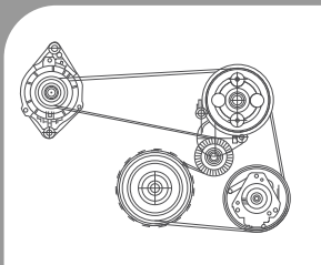
สายพานตัวขับเคลื่อนและคอมเพรสเซอร์ลดเสียงรบกวน
