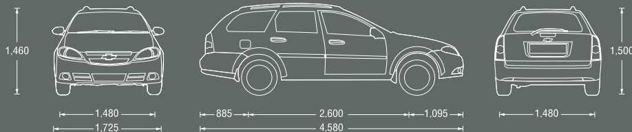
ขนาดตัวรถ (มม.)
